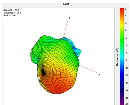
2690MHz
