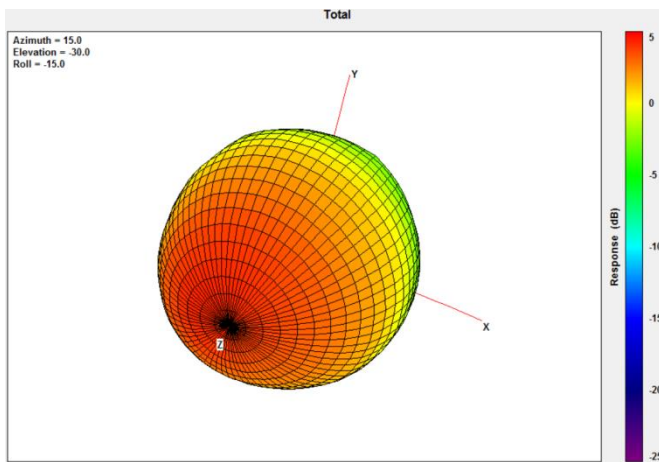
@1575MHz
