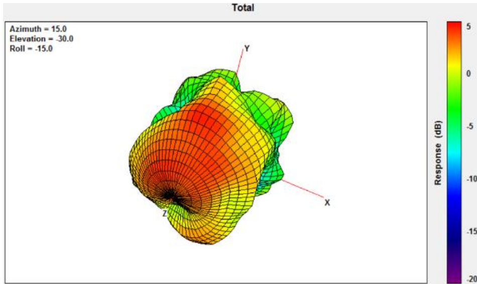
2450MHz
