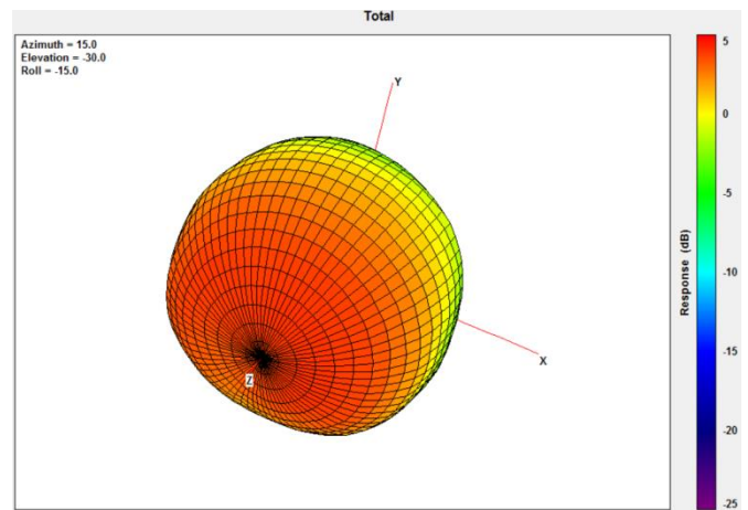
@1602MHz
